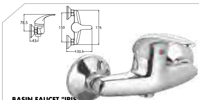
BASIN FAUCET "IRIS" ΜΠΑΤΑΡΙΑ ΜΠΑΝΙΟΥ "IRIS" RUBINETTO A PARETE "IRIS" БАТЕРИЯ ЗА УМИВАЛНИК "IRIS"
