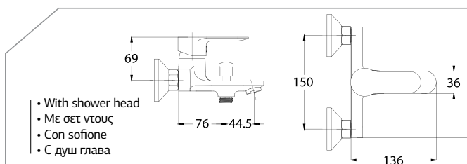
BATHROOM FAUCET "SIERRA" ΜΠΑΤΑΡΙΑ ΜΠΑΝΙΟΥ "SIERRA" RUBINETTO DA BAGNO "SIERRA" БАТЕРИЯ ЗА БАНЯ "SIERRA"
